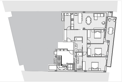
PLANTA PRIMERA
