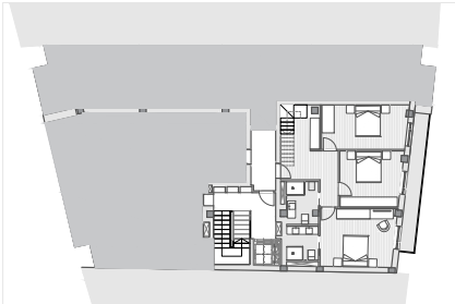
PLANTA CUARTA
