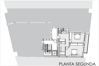
PLANTA SEGUNDA
