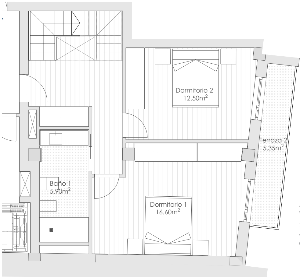
PLANTA SEGUNDA
